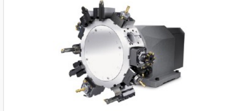
Takım Tutucuları
